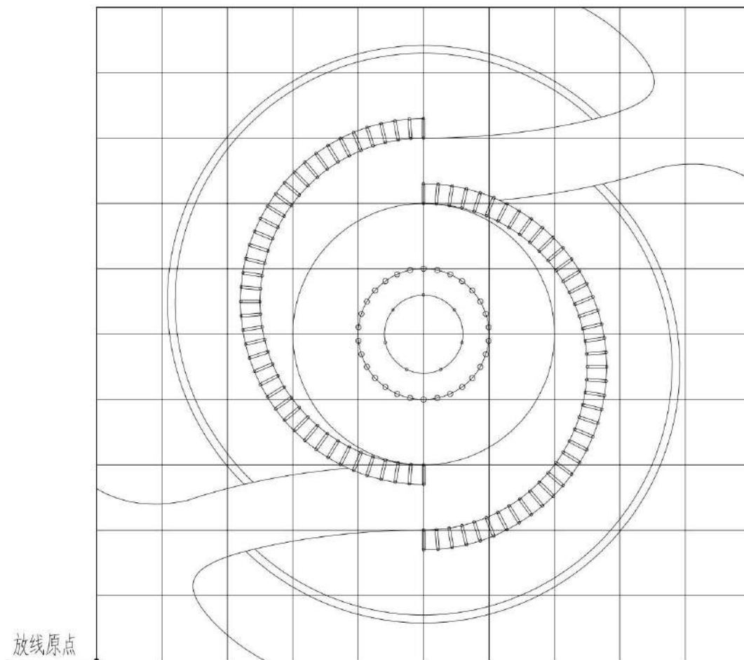
1 总平面网格放线图 SCALE 1:50
