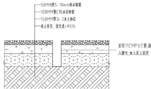
5 垂直状态直径8CM圆竹固定做法
