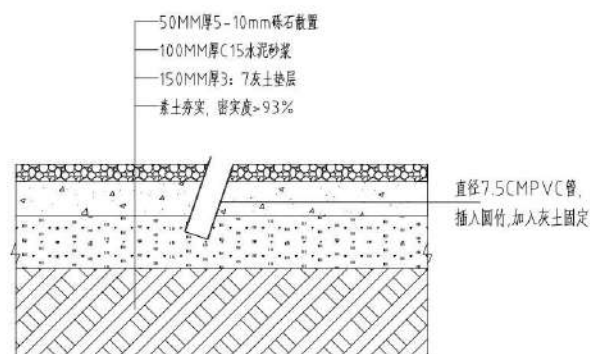
4 倾斜状态直径4CM圆竹固定做法
