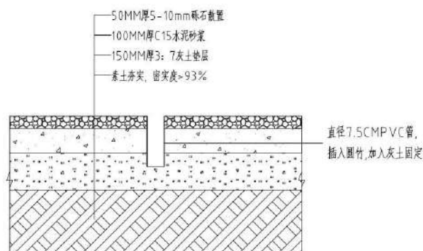
3 垂直状态直径4CM圆竹固定做法
