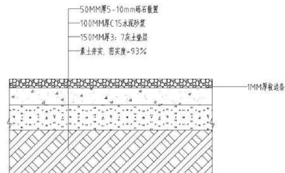
1 砾石铺装做法
