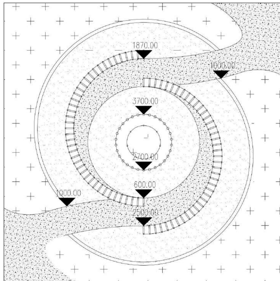
1 总平面图竖向标高图 SCALE 1:50
