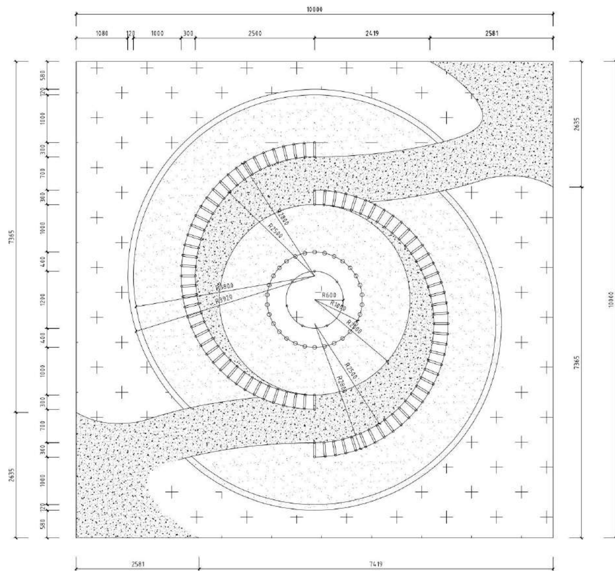
1 总平面尺寸标注图 SCALE 1:50
